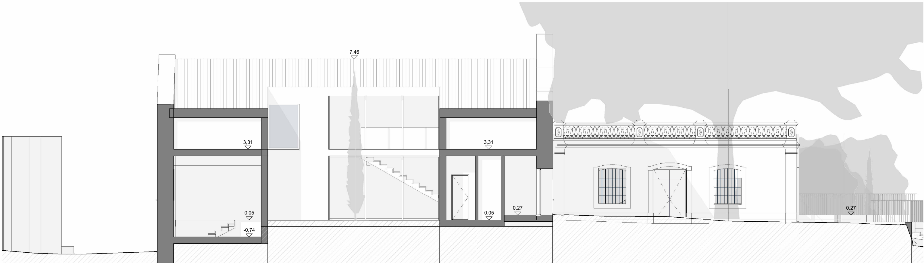
Alçado Este
