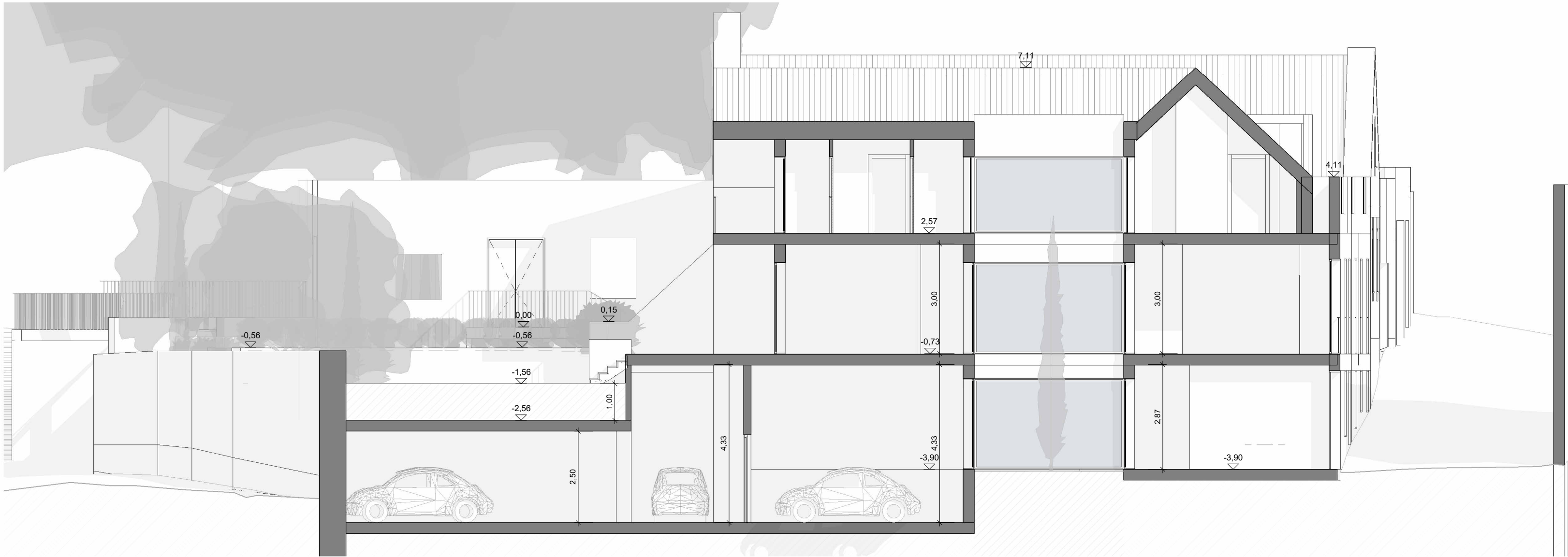
Corte B
