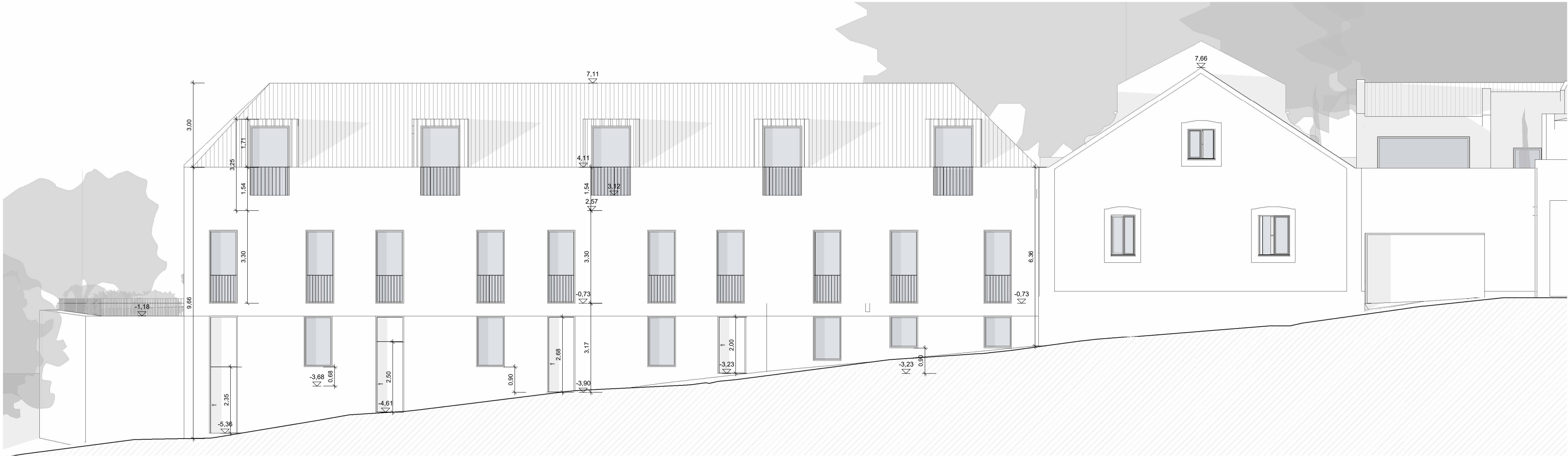
Alçado Sul
